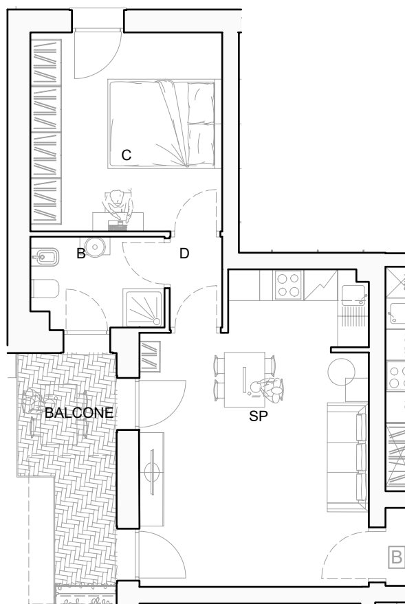
PIANO PRIMO
